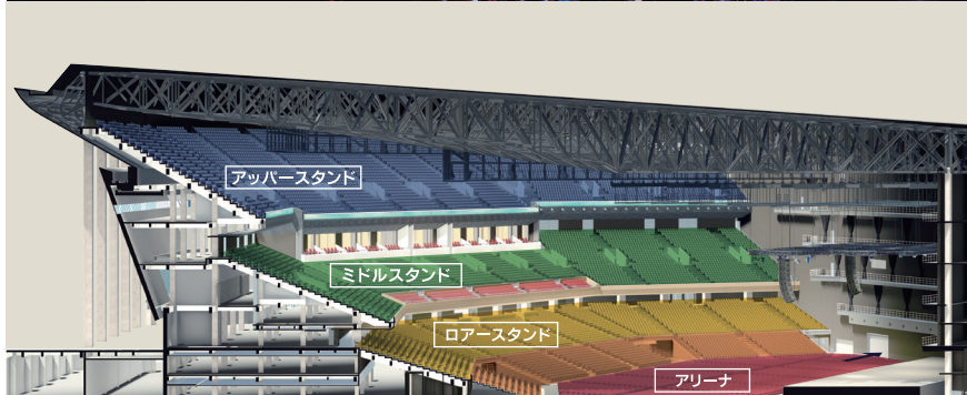
アリーナ断面
